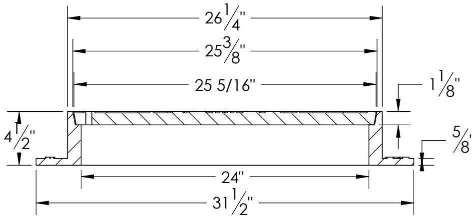
SECTION A-A SCALE 1 : 8
